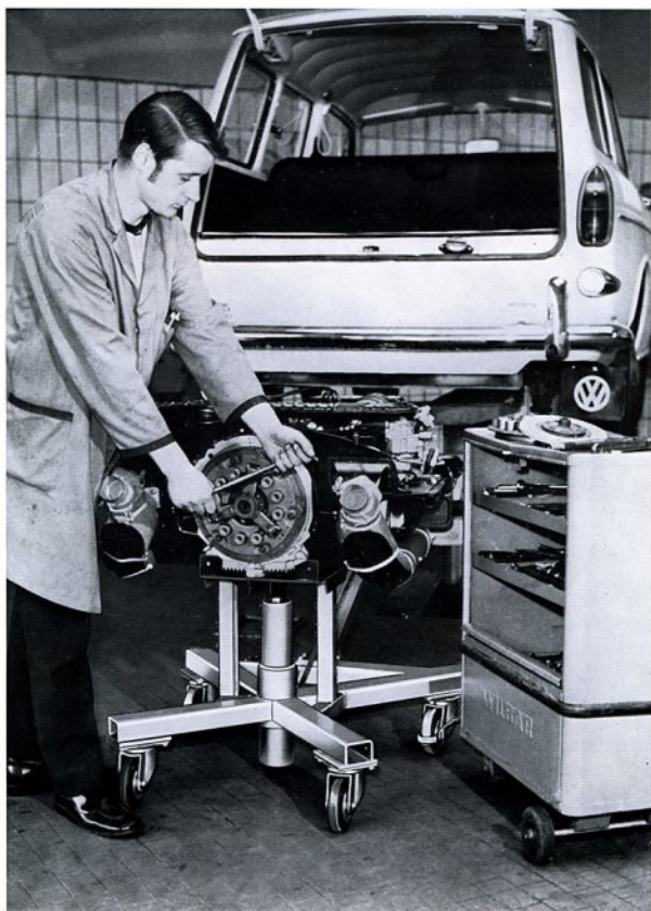
Überholung der Kupplung am Fahrzeug.
